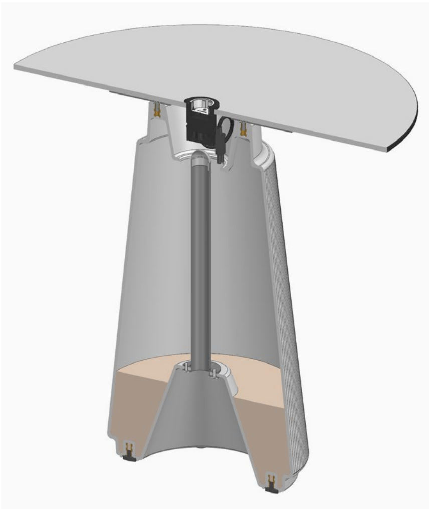
Columna electrificada con un tubo interior fabricado en acero con un diámetro de 40 mm y atornillado a la parte inferior de la columna.
